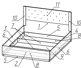
Рис.1 Схема сборки
